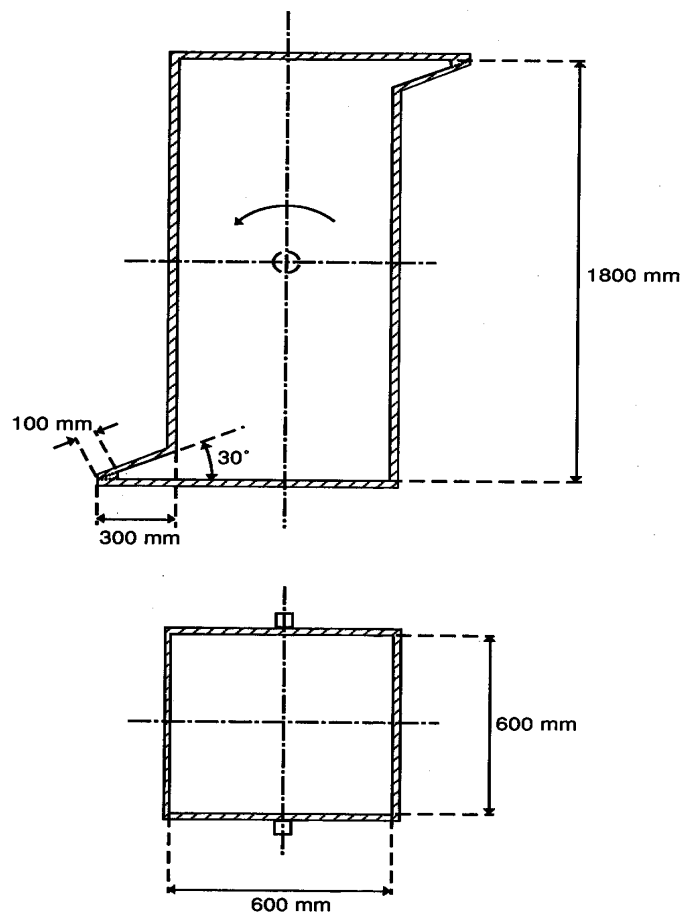
그림 I.1 - 회전충격 시험장치
