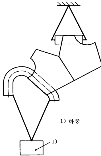
그림 A.3 조끼형 부력기구(수직강도 시험)
