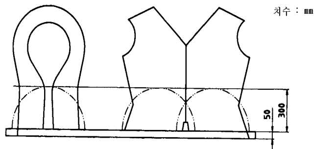
그림 E.1 : 시험편 파지장치
